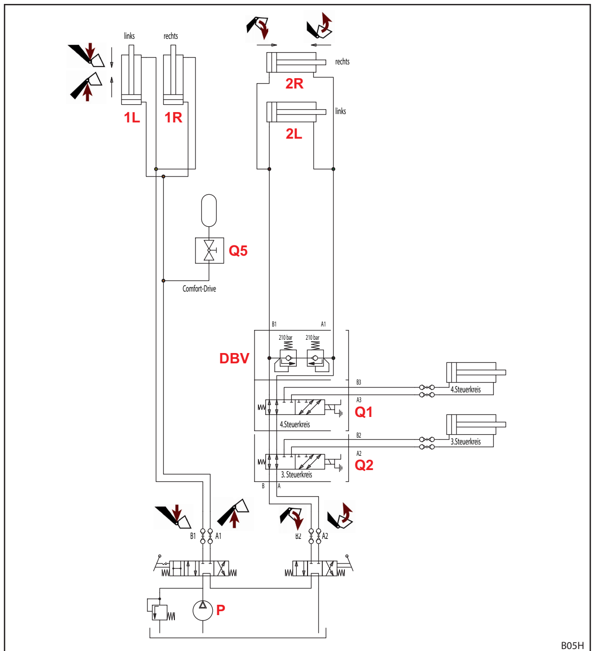
Abb. 126 Hydraulikplan H
