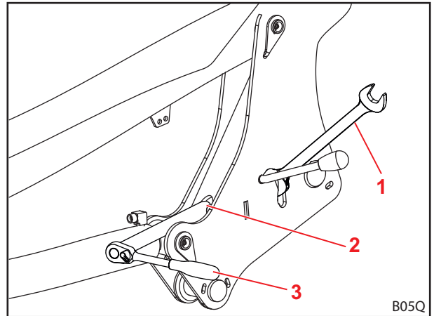
Abb. 61 Werkzeug anlegen
