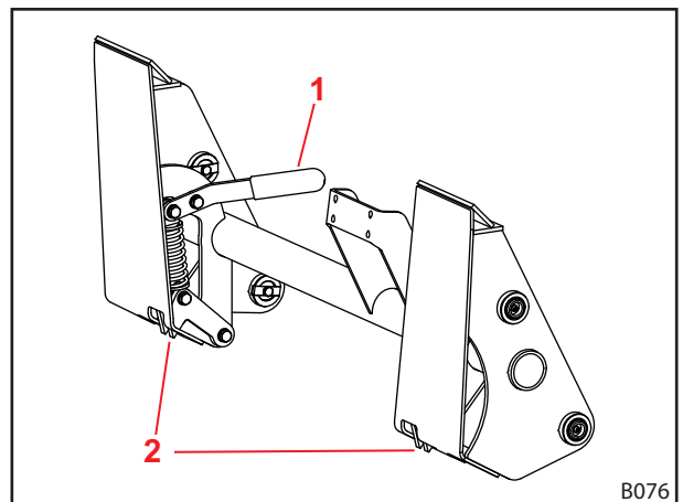
Abb. 87 Werkzeug-Verriegelung am Skid-Steer-Wechselrahmen
