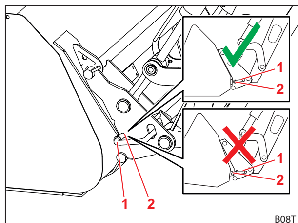
Abb. 85 Position der Verriegelungsbolzen prüfen
