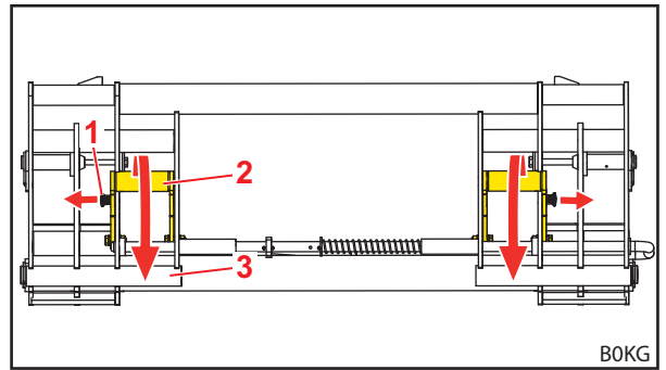
Abb. 89 Anlagen herunterschwenken
