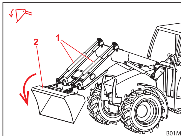
Abb. 31 Schütten-Funktion
