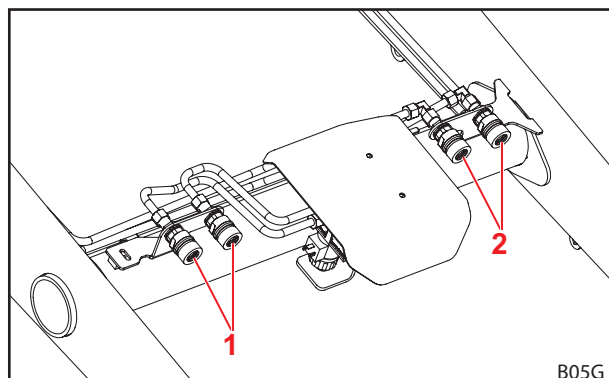
Abb. 46 Zusätzlicher 4. Steuerkreis
