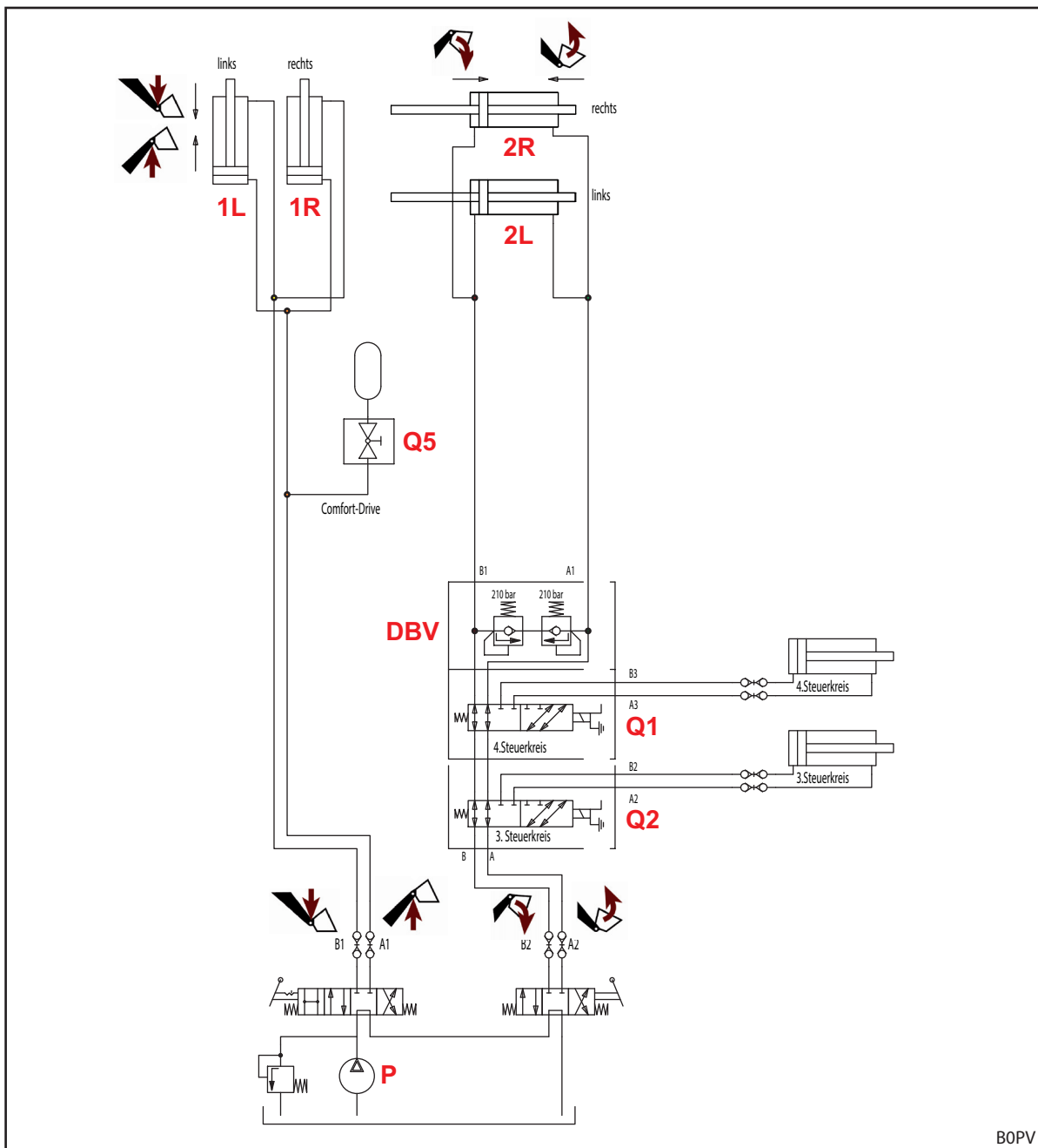
Abb. 127 Hydraulikplan P
