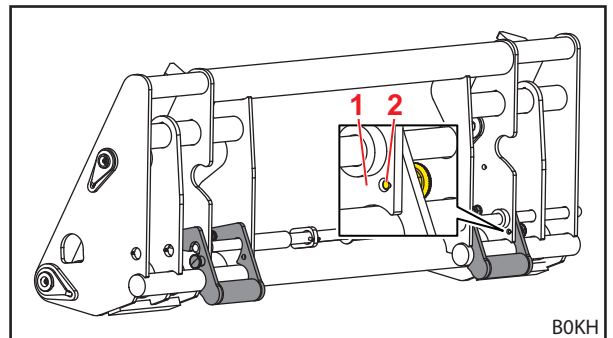
Abb. 90 Heruntergeschwenkte Anlagen
