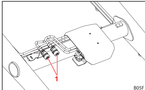
Abb. 45 Zusätzlicher 3. Steuerkreis
