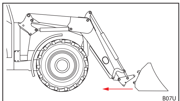
Abb. 108 Wegfahren
