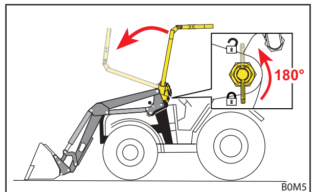
Abb. 36 OPG herunterklappen
