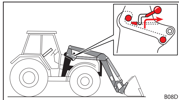
Abb. 122 Frontlader-Verriegelung lösen
