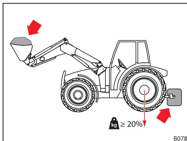
Abb. 50 Belastung bei Frontladerarbeiten
