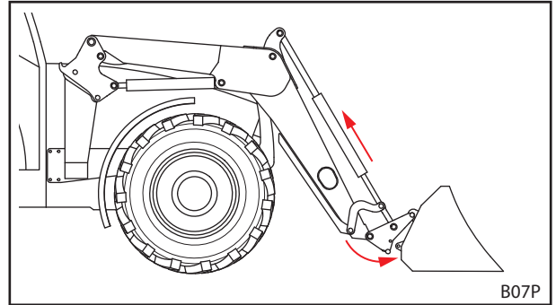
Abb. 98 Einhängen
