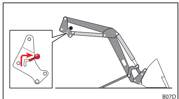
Abb. 53 Frontlader-Verriegelung öffnen
