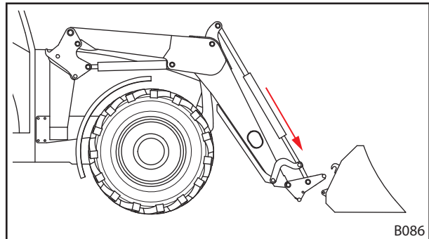
Abb. 96 Schwingen positionieren
