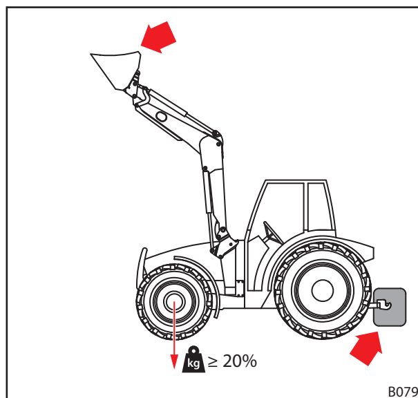
Abb. 51 Belastung bei Straßenfahrten
