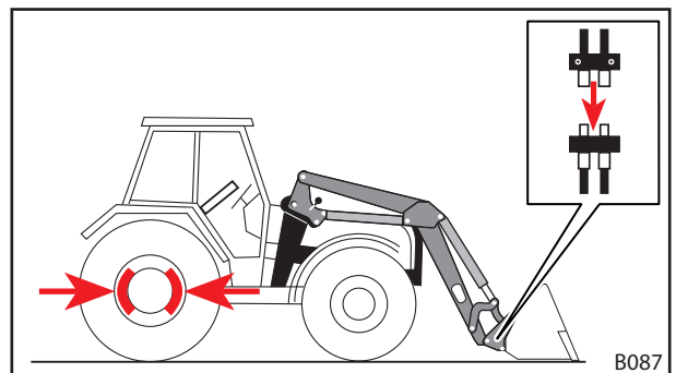
Abb. 100 Hydraulikleitungen des Werkzeuges mit Frontlader-Kupplungen verbinden
