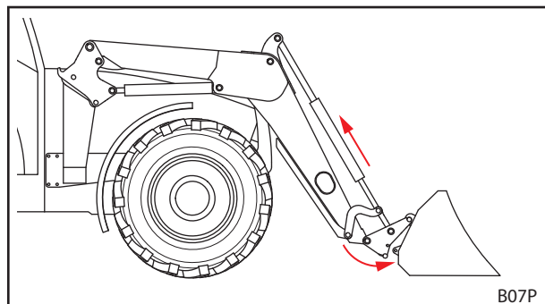
Abb. 103 Einhaken
