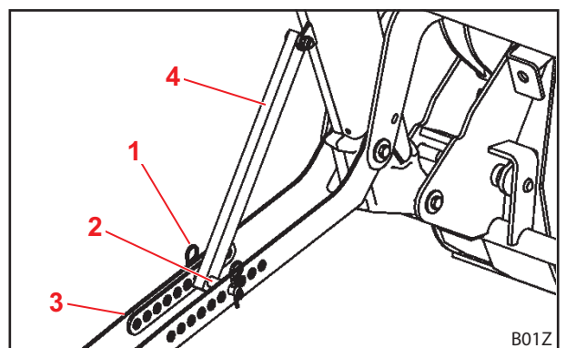
Abb. 78 Abstellstütze
