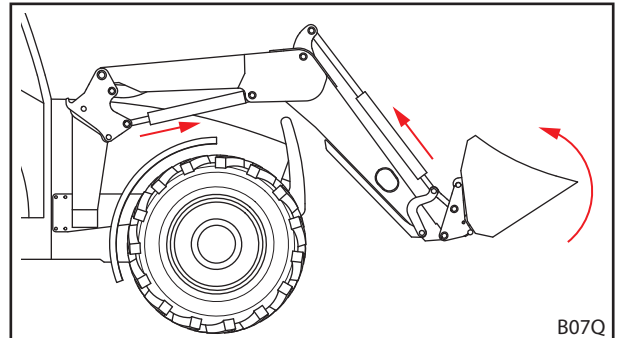
Abb. 99 Werkzeug-Verriegelung auslösen
