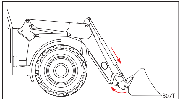
Abb. 107 Wechselrahmen aushaken
