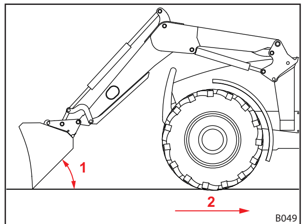
Abb. 109 Rückwärts planieren
