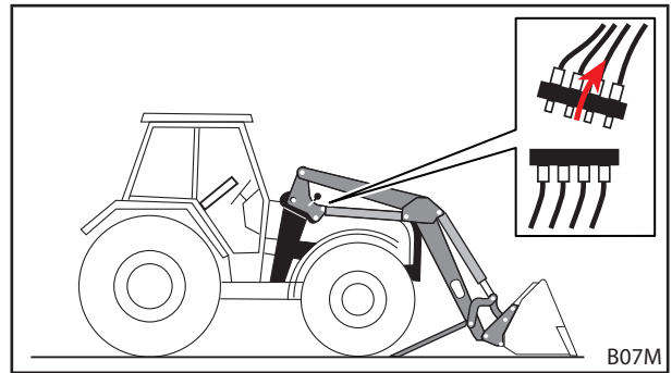
Abb. 124 Hydraulik abkoppeln
