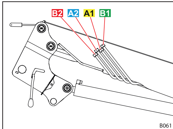
Abb. 22 Hydraulikleitungen
