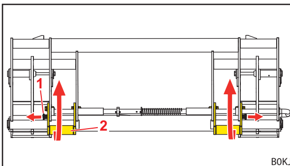
Abb. 91 Anlagen hochschwenken
