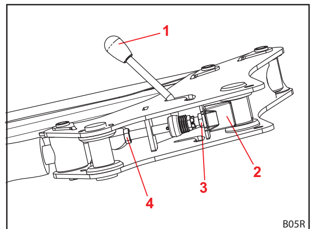
Abb. 63 Ansicht der Frontlader-Verriegelung von unten
