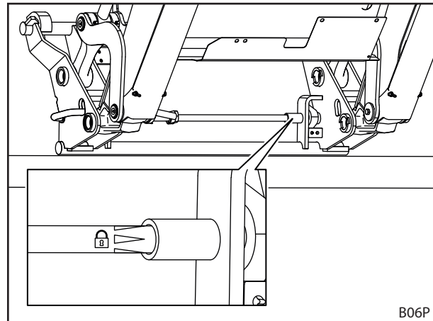
Abb. 83 Werkzeug-Verriegelung anhand des Aufklebers prüfen
