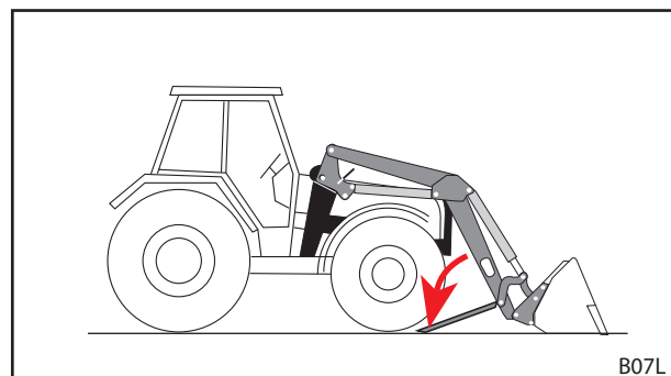
Abb. 123 Abstellstützen ausklappen
