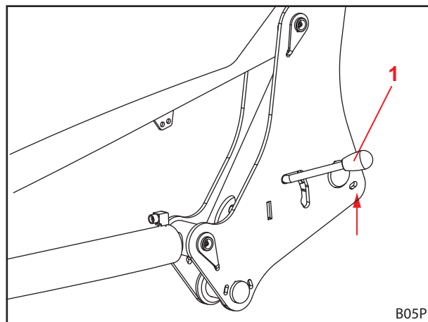
Abb. 119 Frontlader-Verriegelung prüfen
