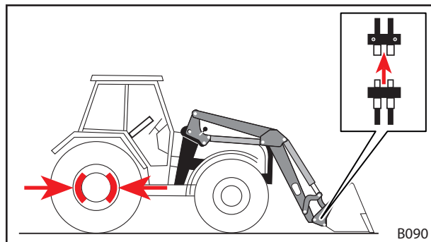
Abb. 106 Hydraulikleitungen lösen
