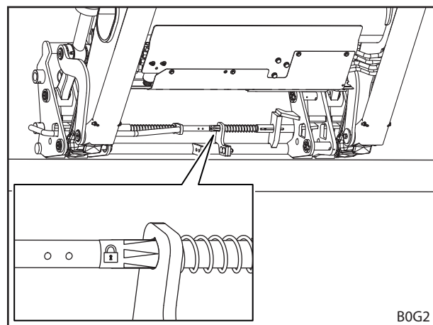
Abb. 84 Werkzeug-Verriegelung anhand des Aufklebers prüfen (Kombi-Wechselrahmen Euro-FR)
