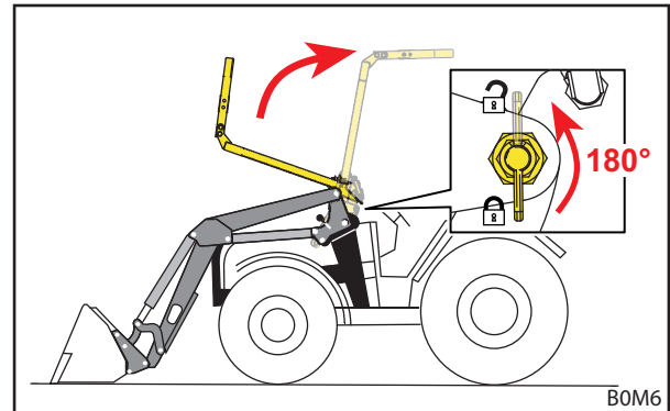
Abb. 38 OPG hochklappen
