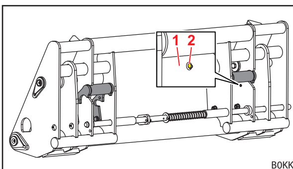
Abb. 92 Hochgeschwenkte Anlagen (Ansicht von hinten)
