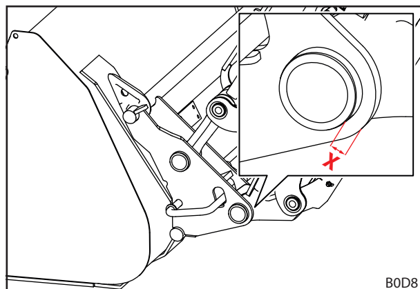
Abb. 120 Verschleißmaß des Wechselrahmens
