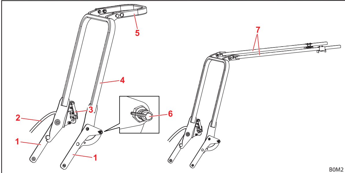
Abb. 11 Operator Protective Guard, OPG, für Traktoren mit hinten angebrachter 2-Pfosten-Umsturzschutzvorrichtung (beispielhafte Abbildung)
