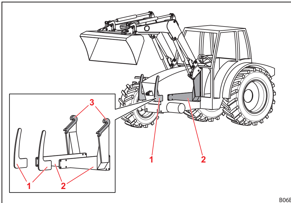
Abb. 13 Anbausatz für Traktor
