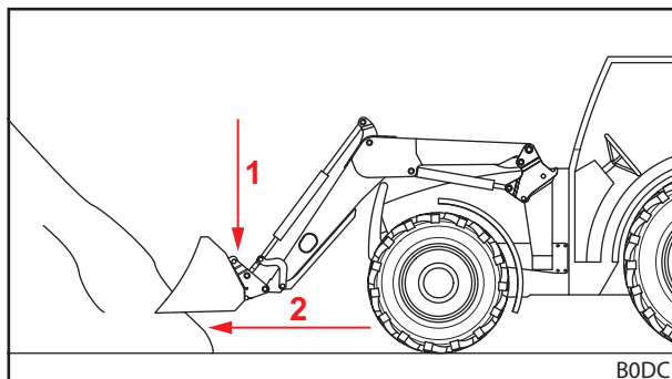
Abb. 98 Frontlader absenken und gerade in Ladegut einfahren
