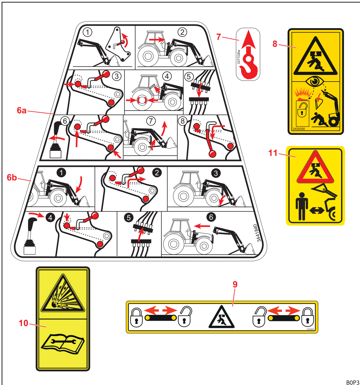
Abb. 6 Sicherheitsaufkleber Position 6-11
