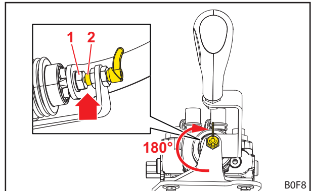
Abb. 63 Verriegelter Bedienhebel
