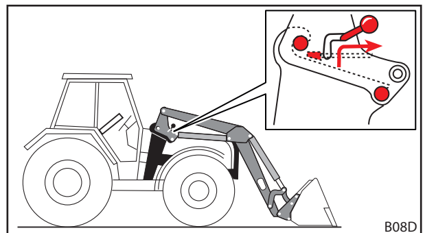
Abb. 107 Frontlader-Verriegelung lösen
