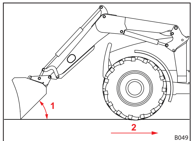
Abb. 96 Rückwärts planieren
