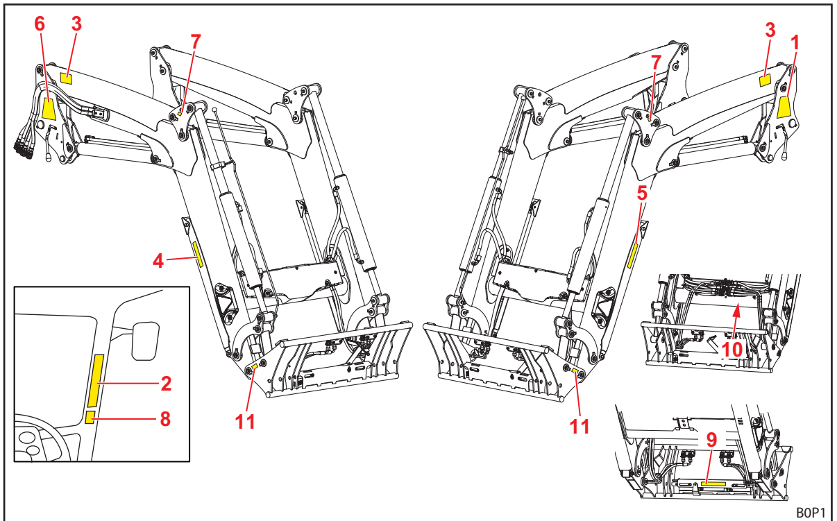
Abb. 4 Frontlader TL (beispielhafte Abbildung)
