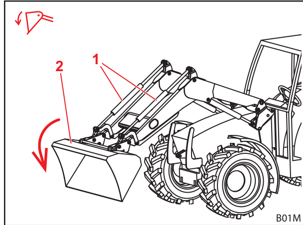
Abb. 25 Schütten-Funktion
