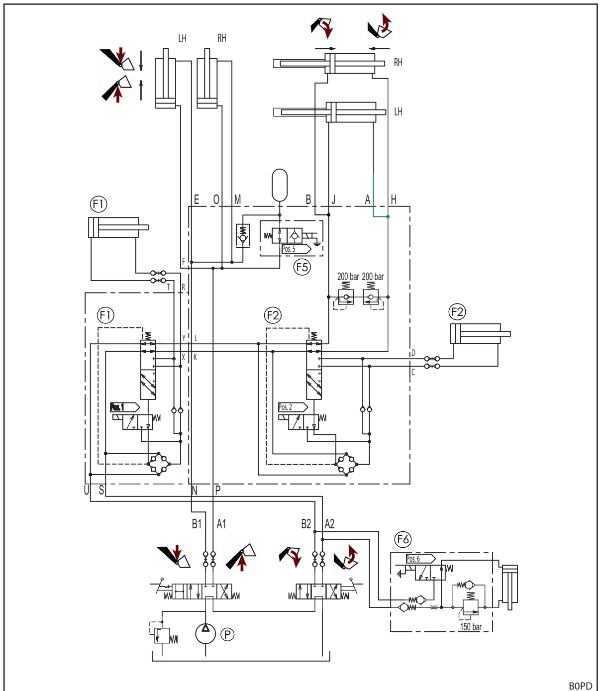
Abb. 112 Hydraulikplan TL
