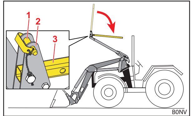
Abb. 36 Heruntergeklappter oberer Bügel
