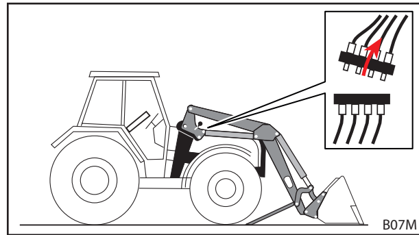
Abb. 109 Hydraulik abkoppeln
