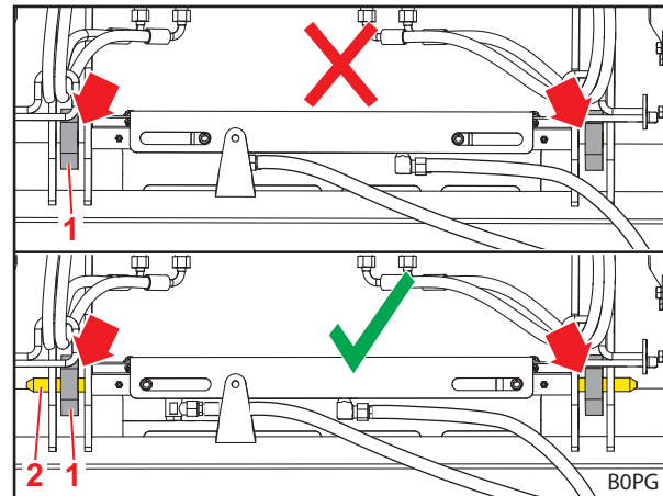
Abb. 82 Position der Verriegelungsbolzen prüfen
