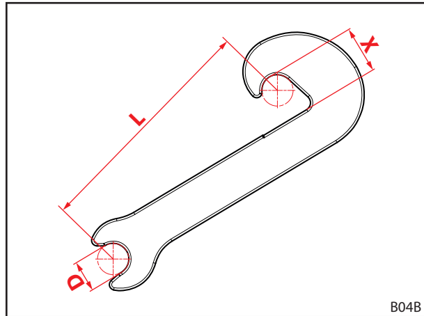
Abb. 104 Verschleißmaße des Fanghakens
