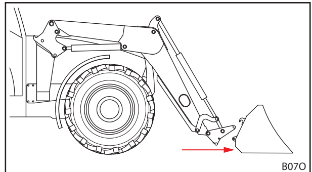
Abb. 90 Heranhfahren
