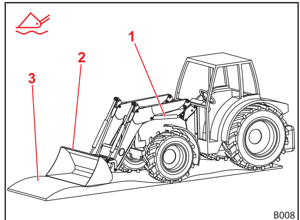
Abb. 26 Frontlader in Schwimmstellung
