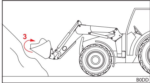
Abb. 99 Werkzeug nach hinten kippen und Ladegut aufnehmen
