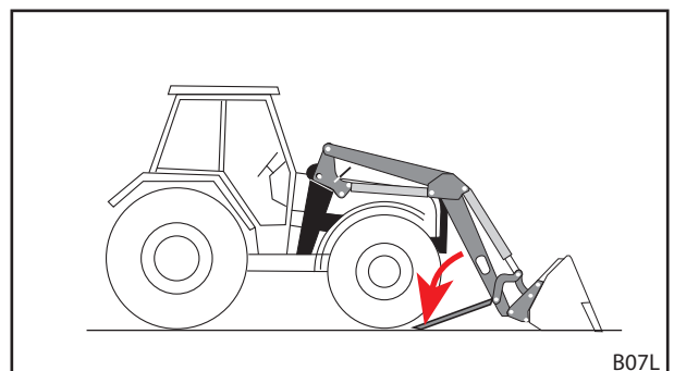
Abb. 108 Abstellstützen ausklappen
