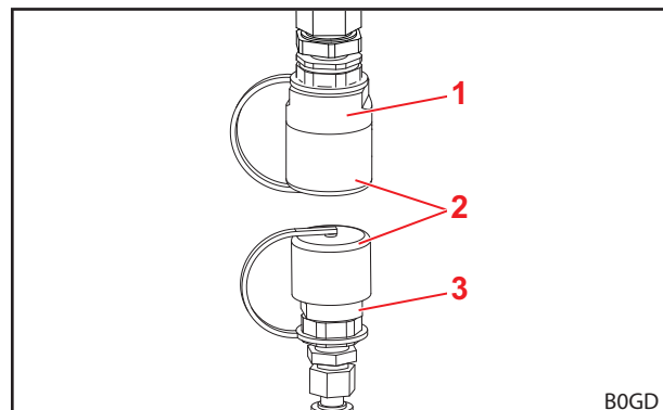
Abb. 73 Schraubkupplungen (beispielhafte Abbildung)
