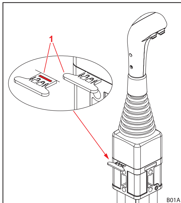
Abb. 59 Verriegelung des Bedienhebels (horizontale Verriegelung)
