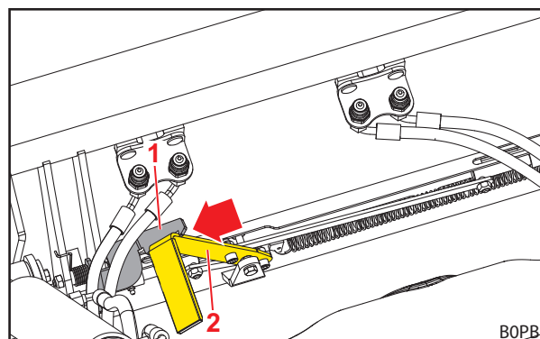
Abb. 84 Geöffnete Werkzeug-Verriegelung
