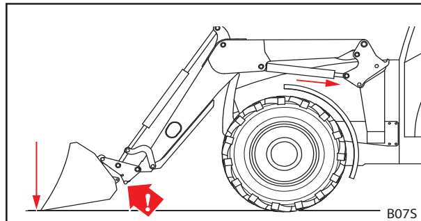
Abb. 79 Werkzeug auf den Boden drücken
