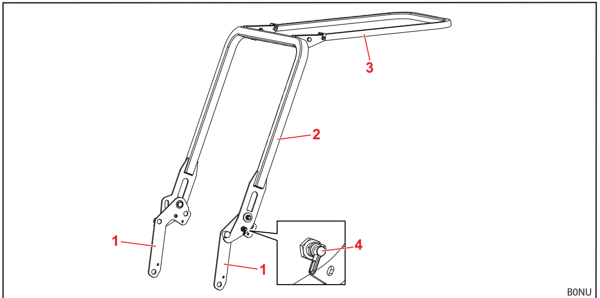
Abb. 12 Operator Protective Guard, OPG, für Traktoren mit vorn angebrachter 2-Pfosten-Umsturzschutzvorrichtung (beispielhafte Abbildung)
