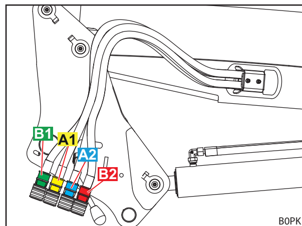
Abb. 15 Hydraulikleitungen
