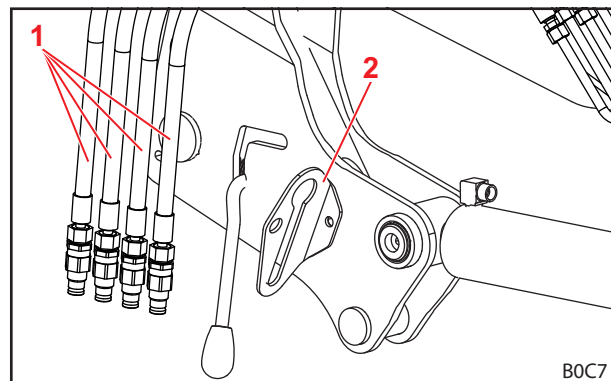
Abb. 111 Hydraulikleitungen in Kupplungshalter einhängen (Darstellung mit Steckkupplungen)
