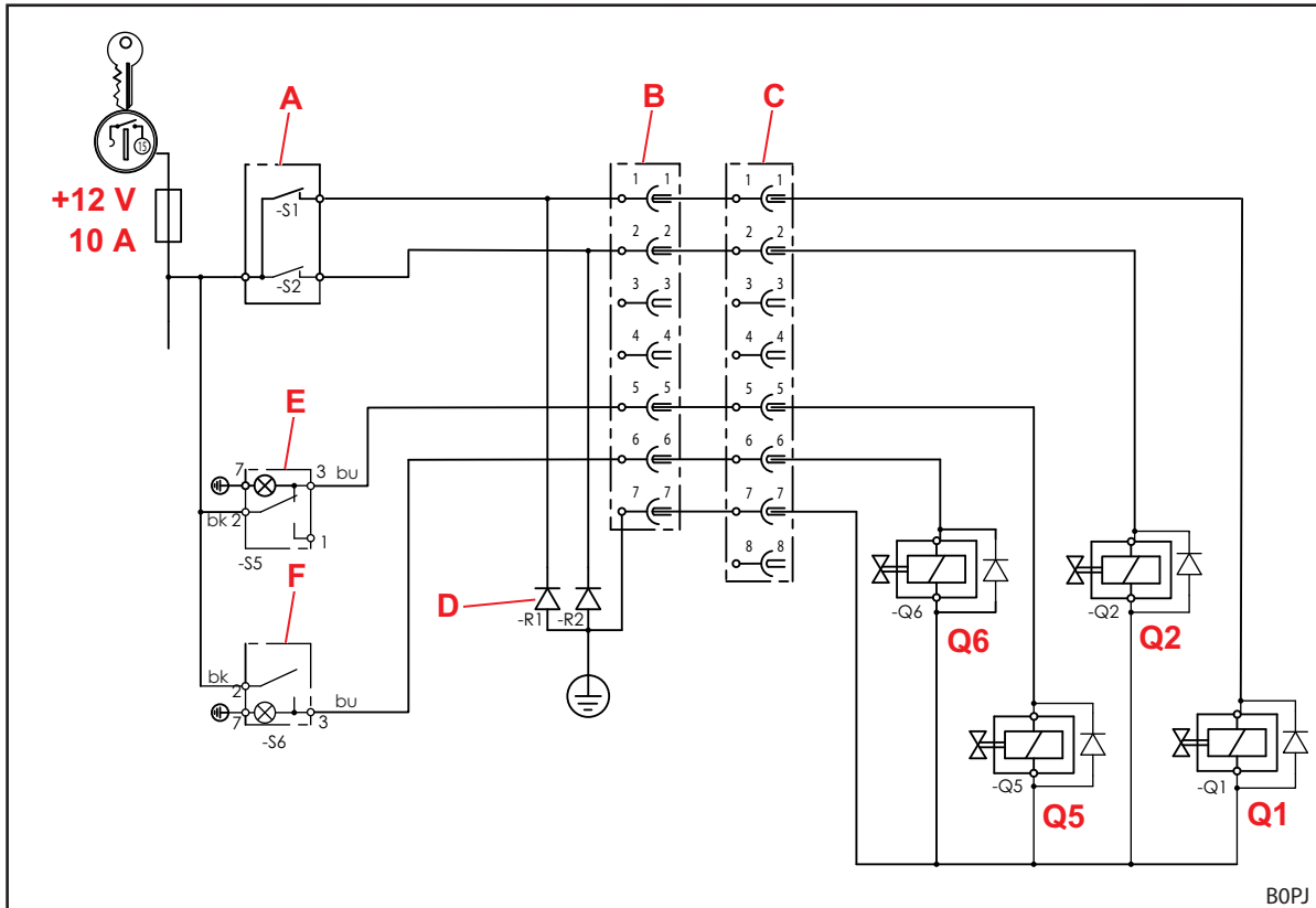
Abb. 113 Elektro-Schaltbild
