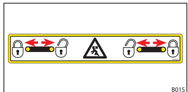
Abb. 81 Position der gelben Indikatoren prüfen
