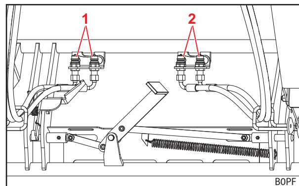
Abb. 39 Zusätzlicher 4. Steuerkreis
