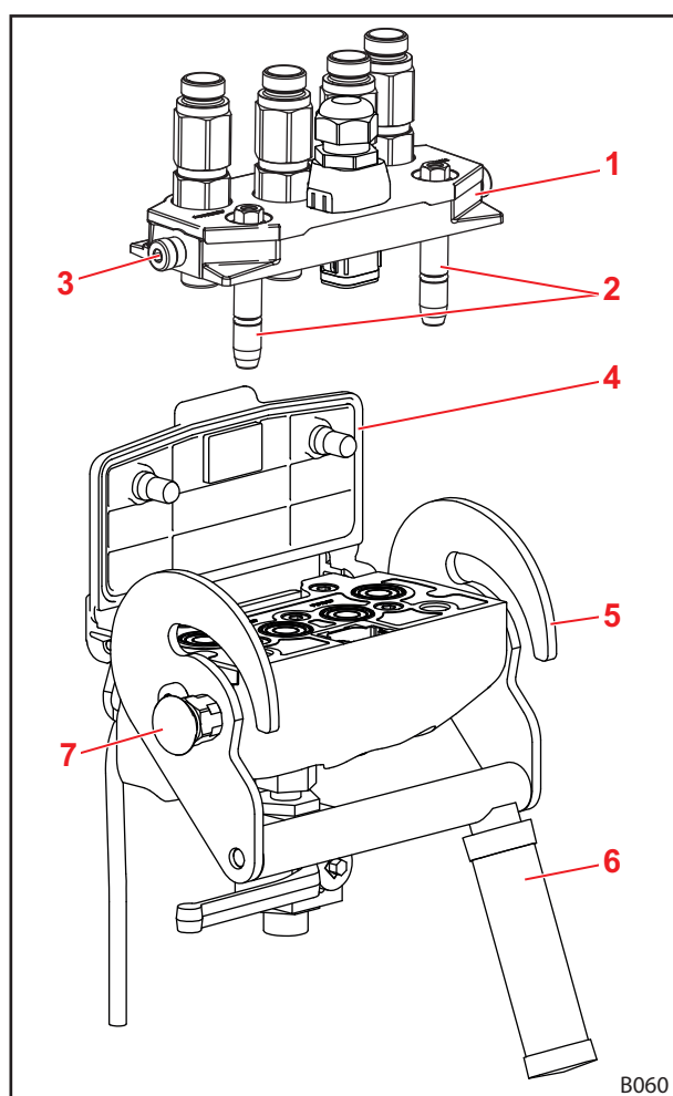
Abb. 74 Hydro-Fix (Beispiel: Hydro-Fix 4-fach)
