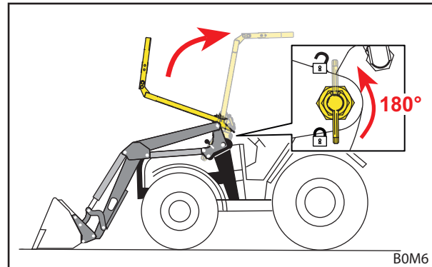
Abb. 31 OPG hochklappen
