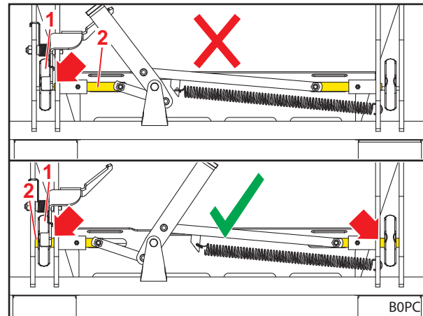
Abb. 78 Position der Verriegelungsbolzen prüfen
