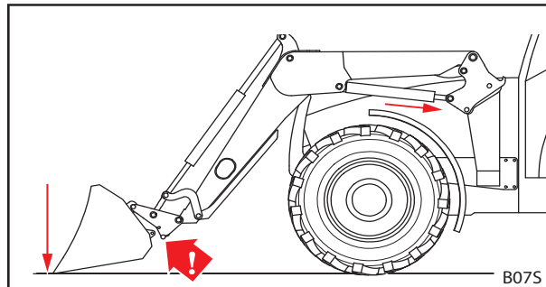
Abb. 83 Werkzeug auf den Boden drücken
