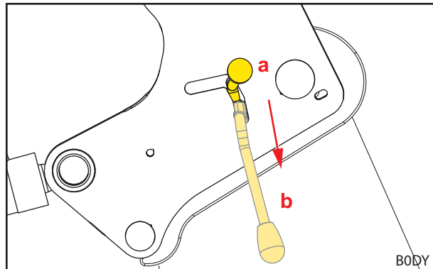
Abb. 54 Spannvorgang des Verriegelungshebels
