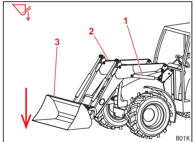
Abb. 23 Senken-Funktion
