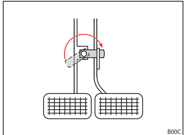
Abb. 41 Bremspedale koppeln
