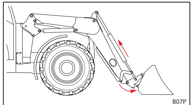
Abb. 91 Einhaken
