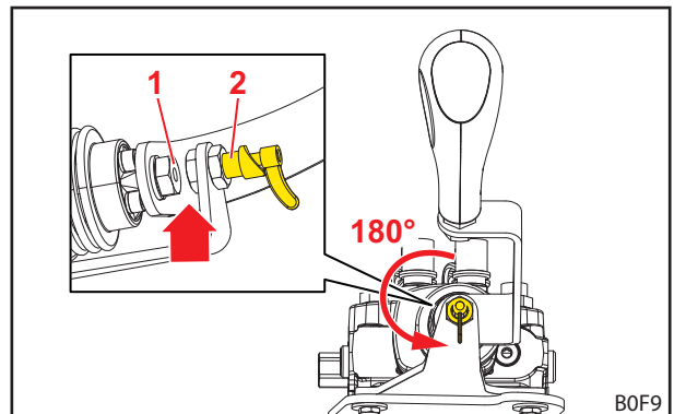
Abb. 64 Entriegelter Bedienhebel
