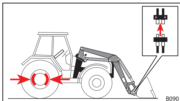
Abb. 93 Hydraulikleitungen lösen
