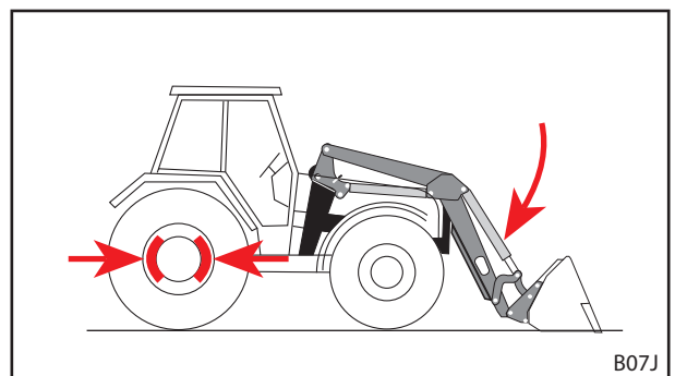
Abb. 106 Feststellbremse anziehen und Frontlader absenken
