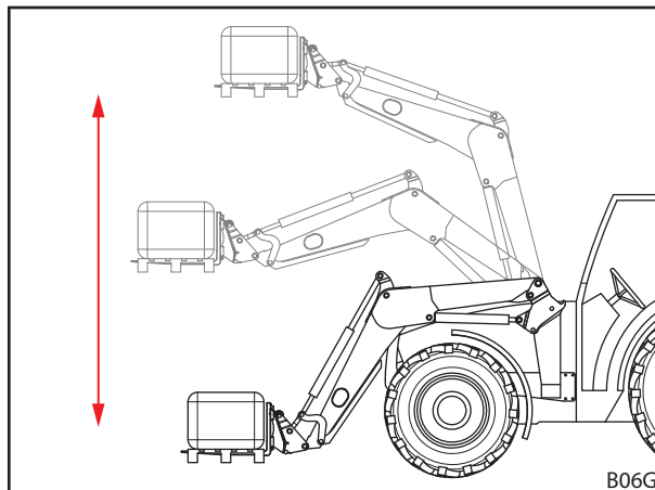
Abb. 28 Mechanische Parallelführung
