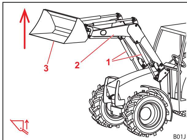
Abb. 22 Heben-Funktion
