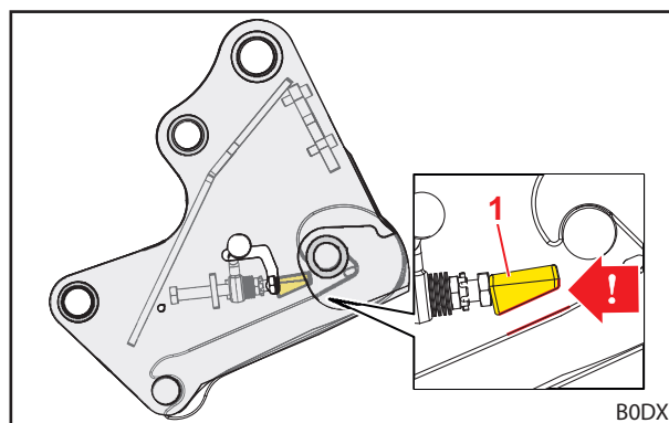
Abb. 51 Korrekte Einbauposition des Klemmkeils
