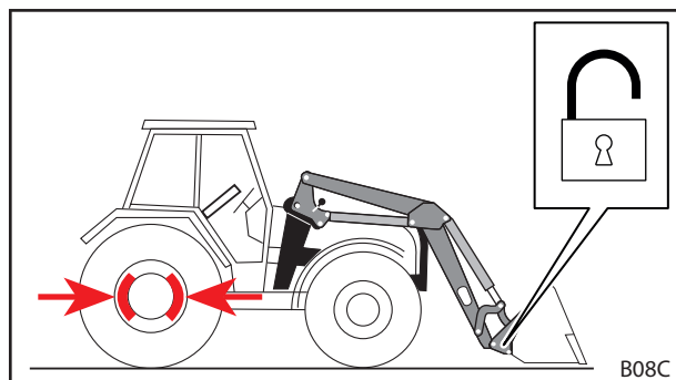
Abb. 92 Werkzeug-Verriegelung öffnen
