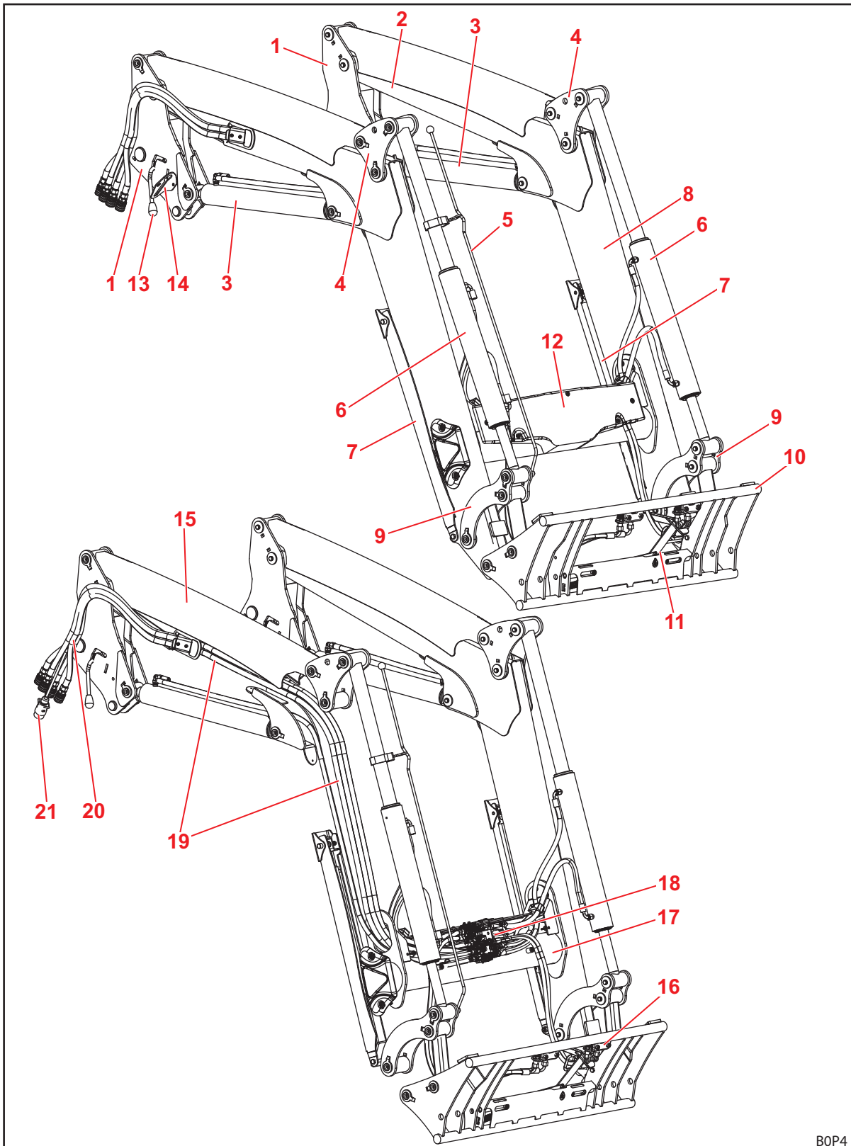
Abb. 10 Frontlader TL
