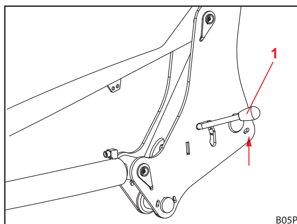
Abb. 52 Frontlader-Verriegelung öffnen
