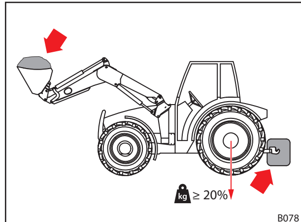
Abb. 42 Belastung bei Frontladerarbeiten
