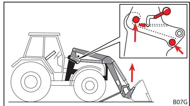
Abb. 49 Heben-Funktion verwenden, bis Frontlader-Bolzen in Fanghaken anliegen
