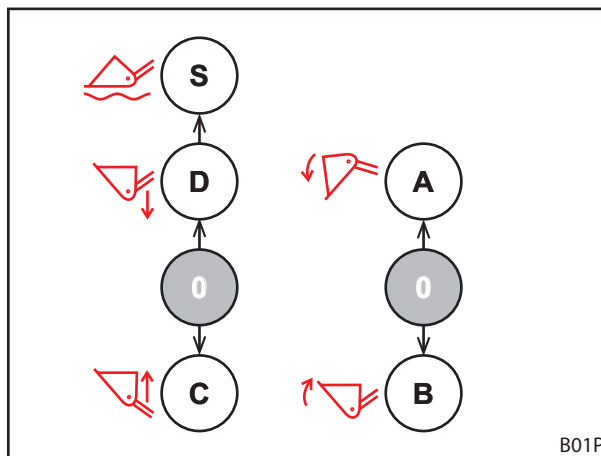
Abb. 57 Belegung bei 2 Bedienhebeln
