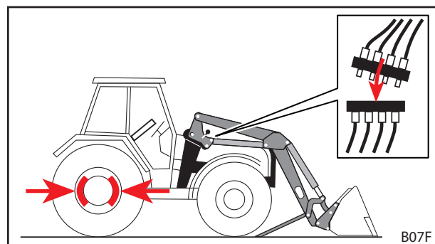
Abb. 47 Traktor abschalten und Hydraulikleitungen anschließen
