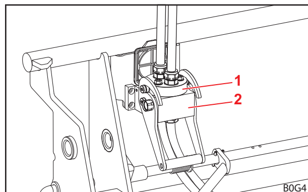
Σχ. 76 Συνδεδεμένη στερέωση εργαλείων
