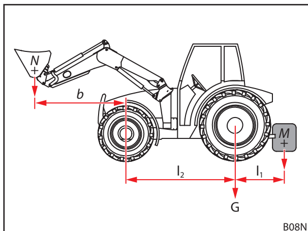
Σχ. 44 Υπολογισμός της στατικής ευστάθειας
