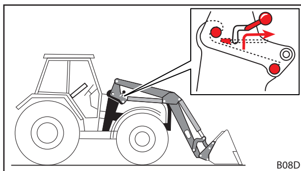
Σχ. 107 Λύσιμο κλειδώματος εμπρόσθιου φορτωτή
