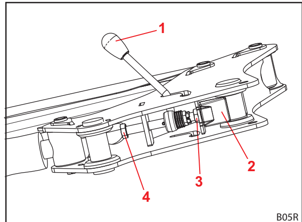
Σχ. 55 Όψη του κλειδώματος του εμπρόσθιου φορτωτή από κάτω
