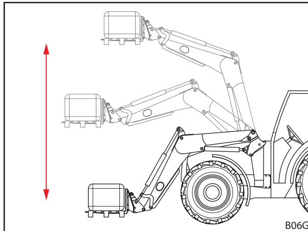
Σχ. 28 Μηχανικός παράλληλος οδηγός
