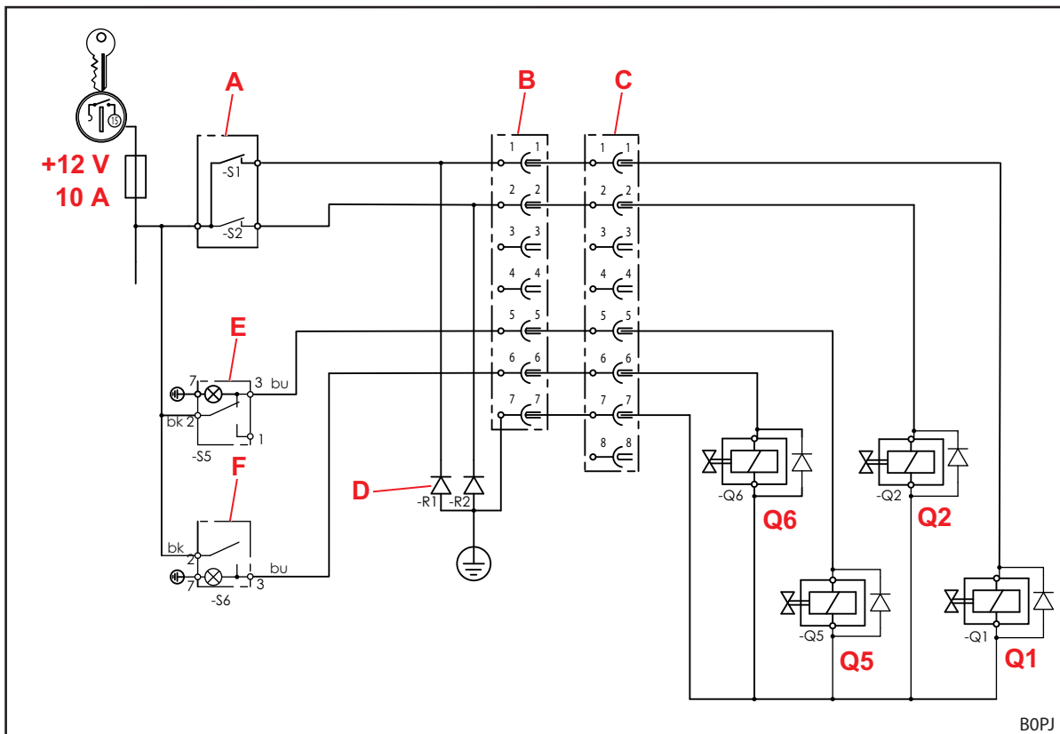
Σχ. 113 Ηλεκτρικό διάγραμμα συνδεσμολογίας
