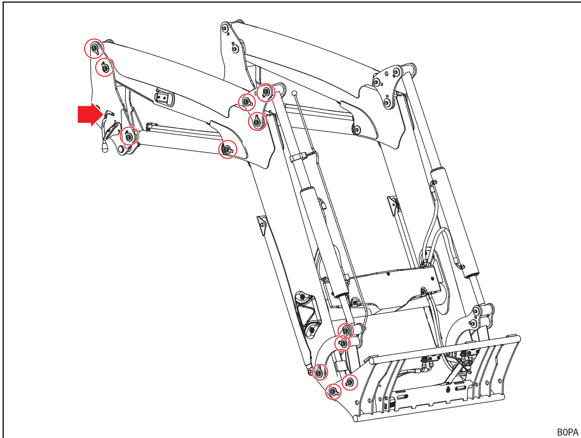
Σχ. 103 Σημεία λίπανσης TL
