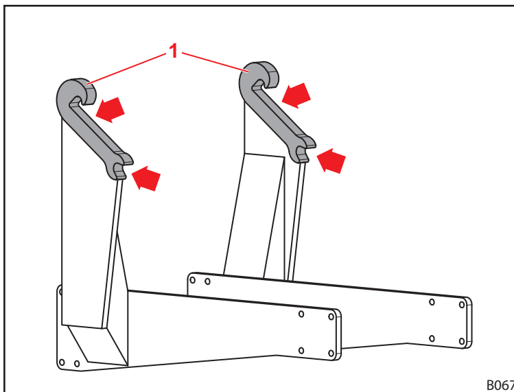
Σχ. 102 Σημεία λίπανσης υποδοχών εμπρόσθιου φορτωτή
