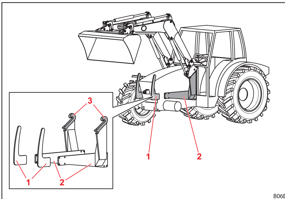
Σχ. 13 Σετ προσάρτησης για τρακτέρ
