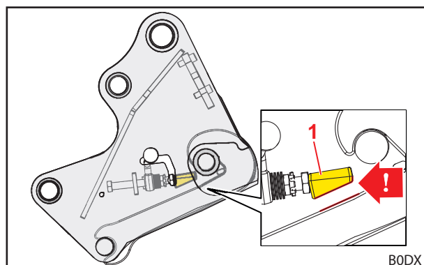
Σχ. 51 Σωστή θέση τοποθέτησης της σφήνας σύσφιξης
