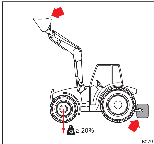
Σχ. 43 Φορτίο σε διαδρομές στον δρόμο
