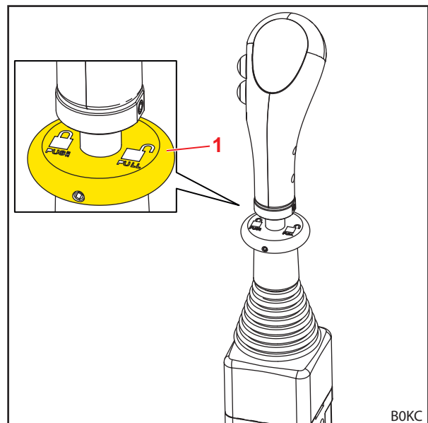
Σχ. 60 Ασφάλιση του μοχλού χειρισμού (κάθετος μηχανισμός ασφάλισης)
