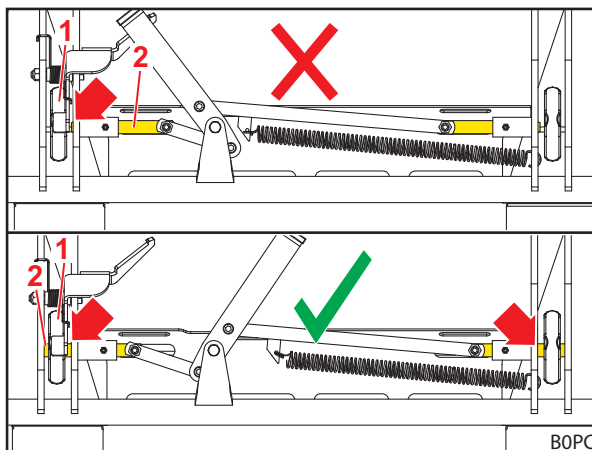
Σχ. 78 Έλεγχος θέσης πείρων ασφάλισης
