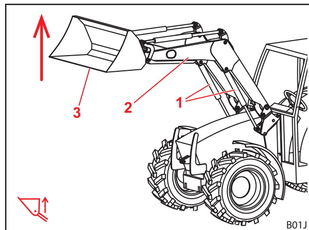
Σχ. 22 Λειτουργία ανύψωσης
