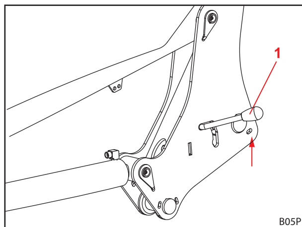
Σχ. 52 Άνοιγμα κλειδώματος εμπρόσθιου φορτωτή
