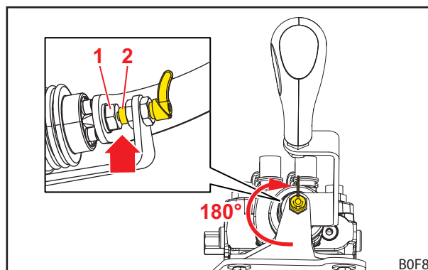
Σχ. 63 Ασφαλισμένος μοχλός χειρισμού
