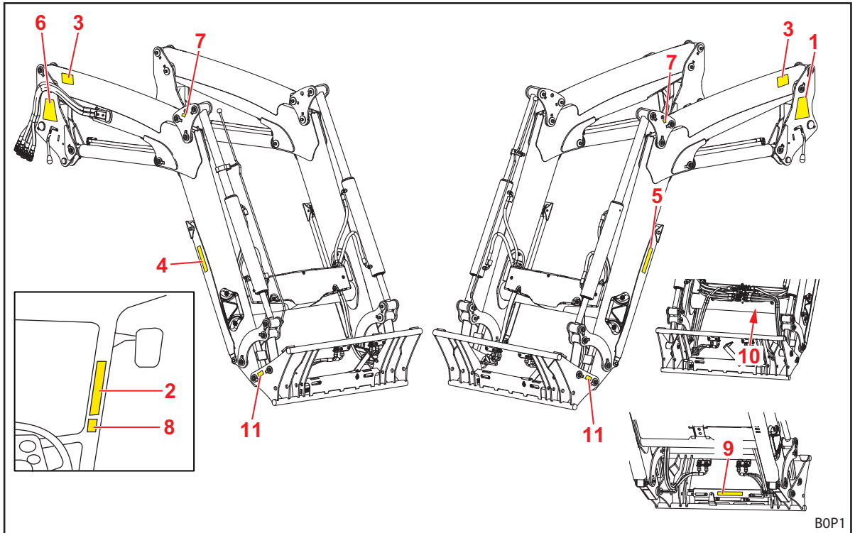
Σχ. 4 Εμπρόσθιος φορτωτής TL (ενδεικτική εικόνα)
