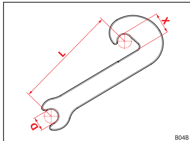
Σχ. 104 Διαστάσεις φθοράς του άγκιστρου
