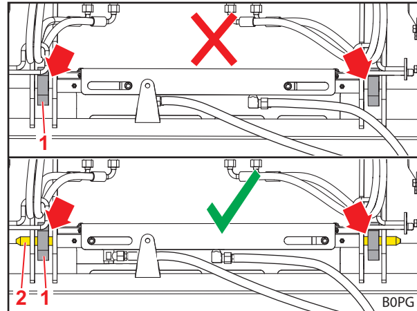
Σχ. 82 Έλεγχος θέσης πείρων ασφάλισης
