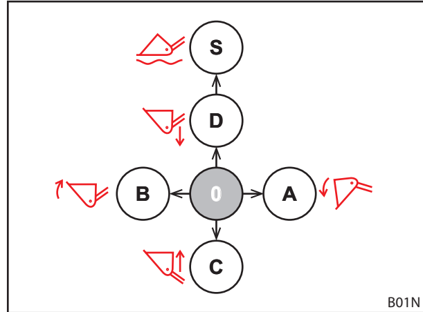
Σχ. 56 Αντιστοίχιση σε έναν μοχλό χειρισμού
