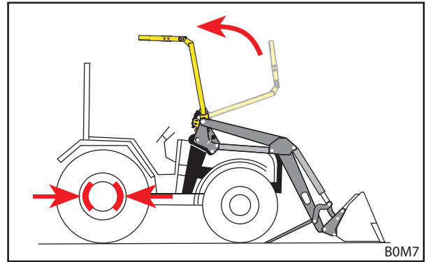
Σχ. 48 Ανέβασμα OPG
