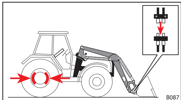
Σχ. 89 Σύνδεση υδραυλικών αγωγών εργαλείου με τους συνδέσμους του εμπρόσθιου φορτωτή
