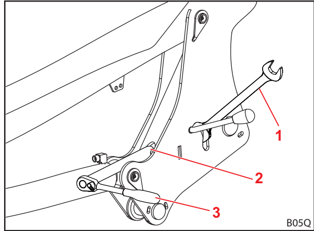
Σχ. 53 Εφαρμογή εργαλείου
