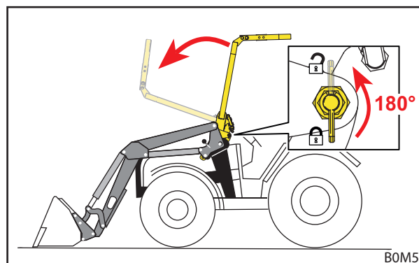
Σχ. 29 Κατέβασμα OPG
