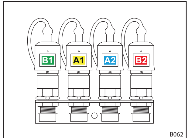
Σχ. 16 Κουμπωτοί σύνδεσμοι συνδεδεμένοι
