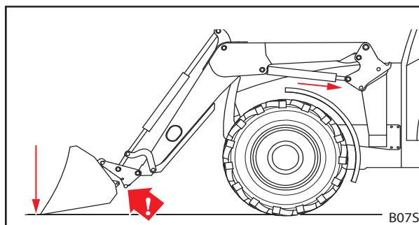
Σχ. 79 Πίεση εργαλείου στο έδαφος
