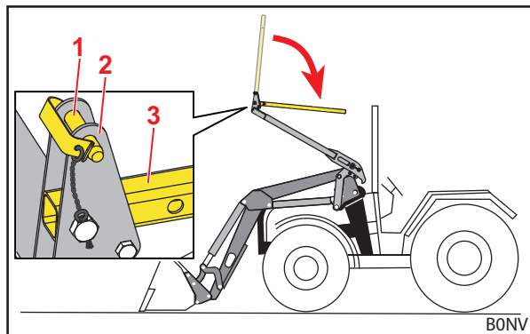
Σχ. 36 Κατεβασμένος επάνω βραχίονας
