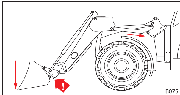
Σχ. 83 Πίεση εργαλείου στο έδαφος
