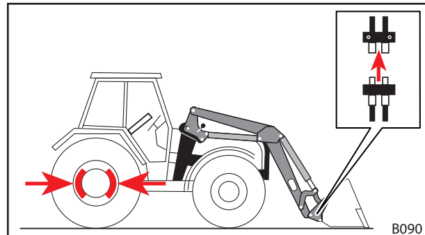
Σχ. 93 Λύσιμο υδραυλικών αγωγών
