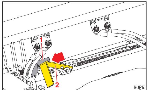
Σχ. 77 Ανοιχτός μηχανισμός ασφάλισης εργαλείου
