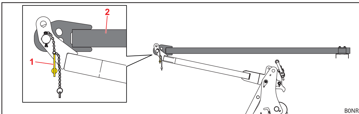
Σχ. 34 Πλήρως κατεβασμένες τραβέρσες
