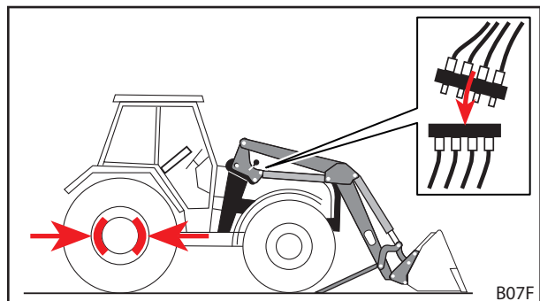
Σχ. 47 Απενεργοποιήστε το τρακτέρ και συνδέστε τους υδραυλικούς αγωγούς
