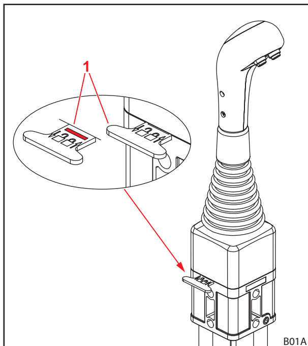
Σχ. 59 Ασφάλιση του μοχλού χειρισμού (οριζόντιος μηχανισμός ασφάλισης)
