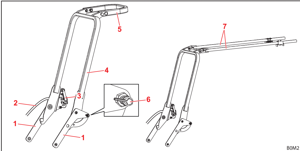
Σχ. 11 Operator Protective Guard, OPG, για τρακτέρ με πίσω τοποθετημένη διάταξη προστασίας από ανατροπή 2 κολονών (ενδεικτική εικόνα)
