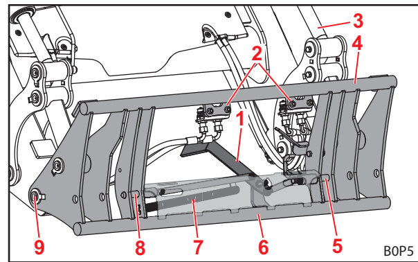
Σχ. 14 Πλαίσιο εναλλαγής Euro
