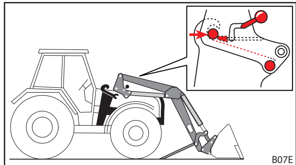
Σχ. 46 Εισαγωγή τρακτέρ στον περιστροφικό βραχίονα
