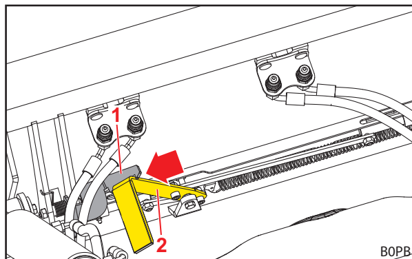
Σχ. 84 Ανοικτός μηχανισμός ασφάλισης εργαλείου
