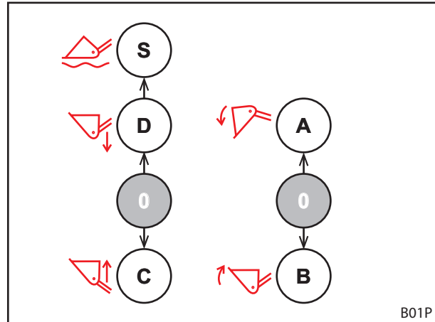
Σχ. 57 Αντιστοίχιση σε 2 μοχλούς χειρισμού
