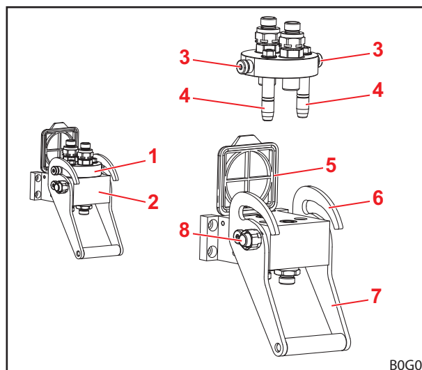
Σχ. 20 Διάταξη στερέωσης εργαλείων
