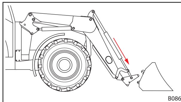
Σχ. 85 Ρύθμιση θέσης περιστροφικού βραχίονα
