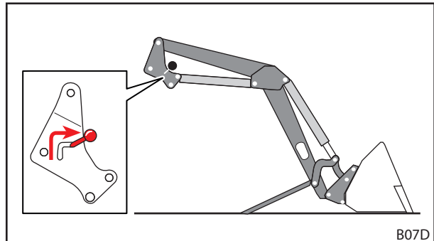
Σχ. 45 Ανοίγμα κλειδώματος εμπρόσθιου φορτωτή
