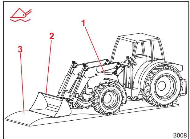
Σχ. 26 Εμπρόσθιος φορτωτής σε θέση πλεύσης
