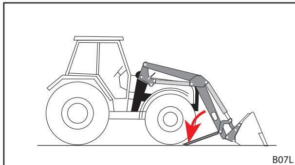
Σχ. 108 Άνοιγμα στηριγμάτων στάθμευσης
