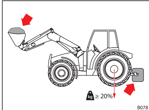
Σχ. 42 Φορτίο σε εργασίες με τον εμπρόσθιο φορτωτή
