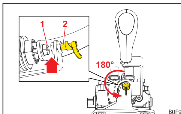
Σχ. 64 Απασφαλισμένος μοχλός χειρισμού
