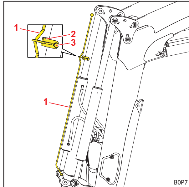
Σχ. 27 Οπτική ένδειξη για τη θέση του εργαλείου
