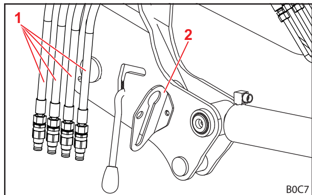
Σχ. 111 Αναρτάτε τους υδραυλικούς αγωγούς στη βάση συνδέσμου (απεικόνιση με κουμπωτούς συνδέσμους)
