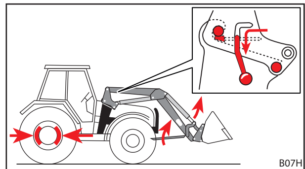
Σχ. 50 Κλείσιμο στηριγμάτων στάθμευσης και κλείσιμο κλειδώματος εμπρόσθιου φορτωτή
