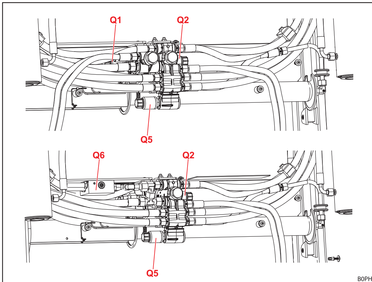
Σχ. 114 Διάταξη υδραυλικών βαλβίδων για πρόσθετες λειτουργίες
