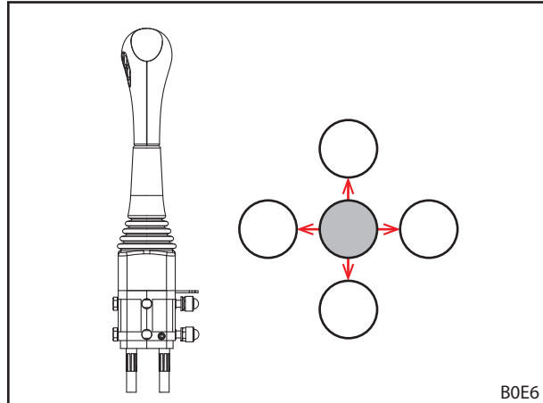
Σχ. 61 Μετακίνηση μοχλού χειρισμού σε όλες τις θέσεις τερματισμού
