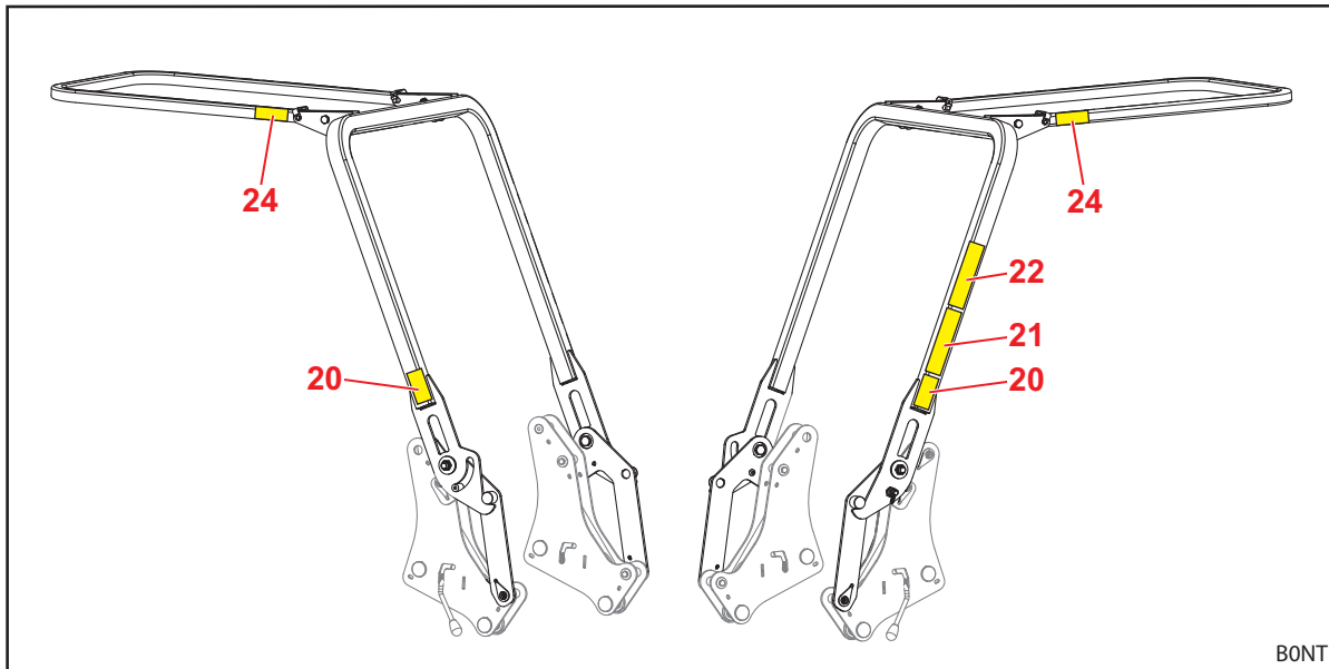
Σχ. 8 OPG για τρακτέρ με μπροστά τοποθετημένη διάταξη προστασίας από ανατροπή 2 κολονών (ενδεικτική εικόνα)
