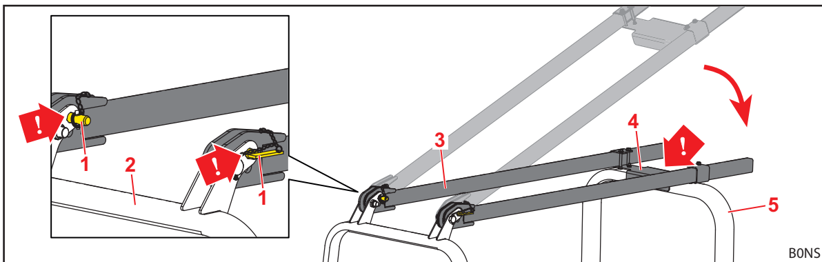
Σχ. 35 Κατεβασμένες και ασφαλισμένες στις επάνω οπές τραβέρσες
